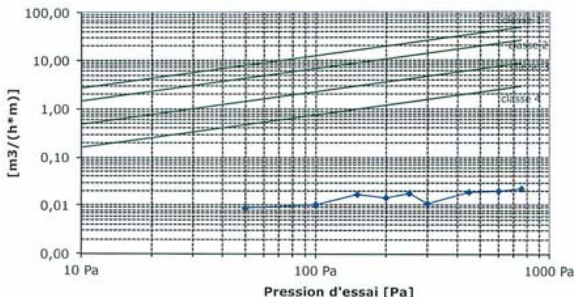
Graphique 1: Perméabilité à l'air relative à la longueur (membrane de largeur 75 mm/100 mm; largeur du joint 30 mm) et les limites supérieures de classes selon DIN EN 12207.
